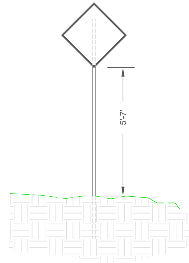
PROFILE SCALE: 3/8" = 1'-0"
